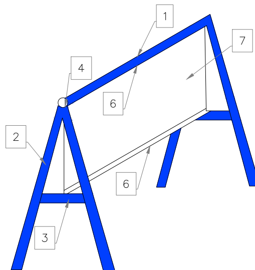
VISTA ISOMÉTRICA
